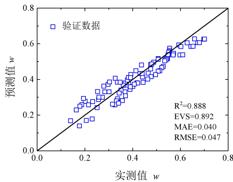
图 5 LightGBM 预测验证数据
