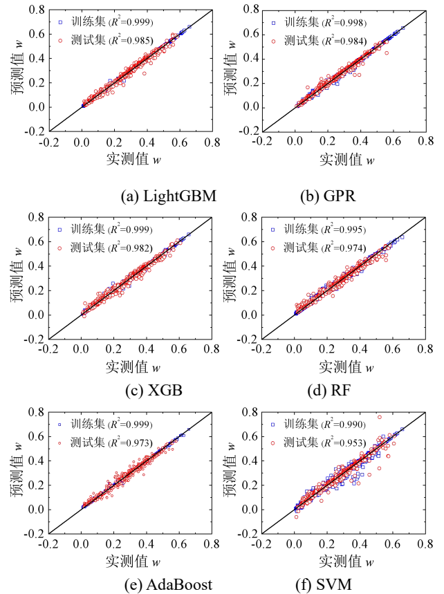
图 2 基于压力水头对数形式下六种算法的预测值与实测值对比
